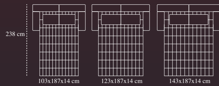
Rete elettrosaldata e materasso a molle con spessore cm. 14
